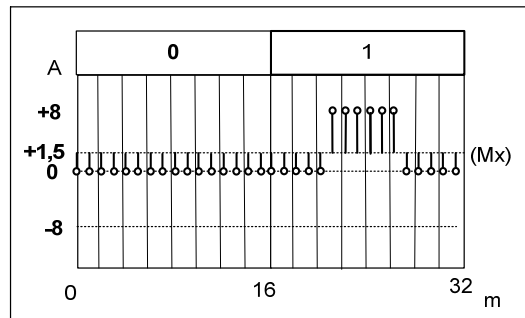
Рис. 5. Центровані значення RZ-сигналу
