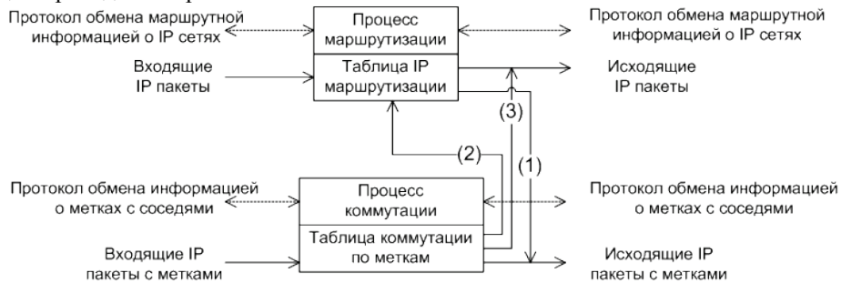
Рис. 12. Взаимосвязь процессов MPLS-коммутации и IP-маршрутизации на LSR / PE-LSR в сетях MPLS
