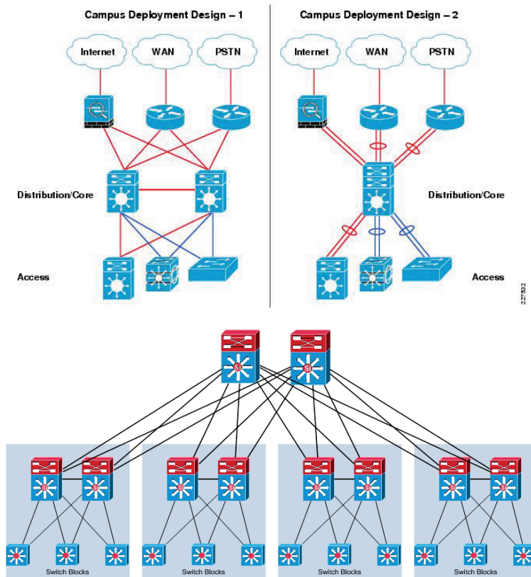
Рис. 2. 2-х рівневе представлення моделі ієрархічної мережі [Core/Distribution-Access — Campus Network по класифікації Cisco Systems Inc.] [5, 6]
