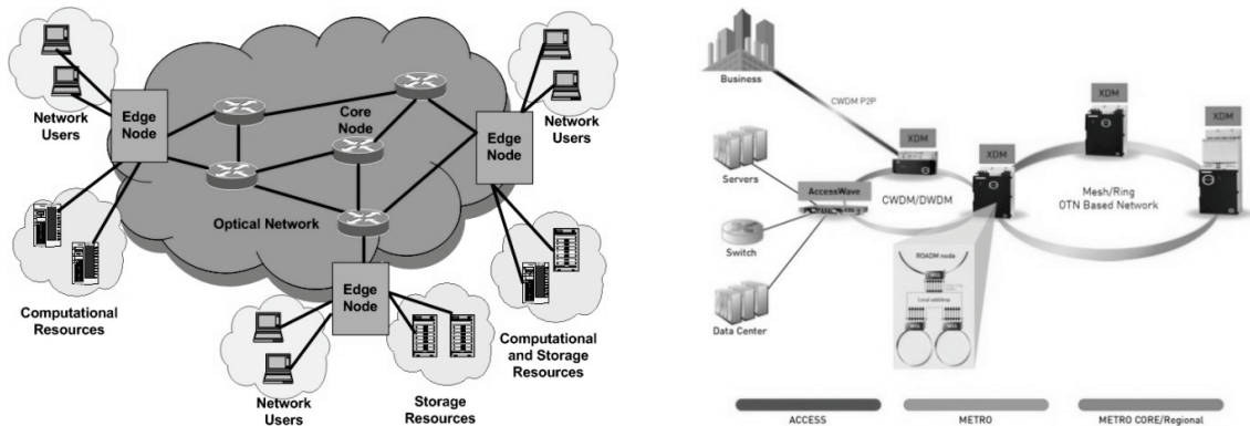
Рис.13. Структура современной корпоративной иерархической оптической информационной сети с ядром
