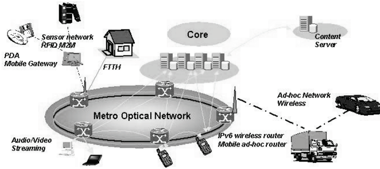
Рис. 14. Различные структурные модели современных иерархических оптических сетей реализованных в мире на базе архитектуры Enterprise Campus Architecture Network (Core-Distribution-Access, CDA) на базе современных стандартов ATM, SDH, SONET и MPLS
