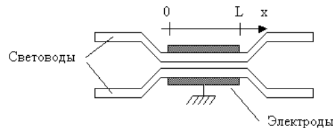
Рис. 16. Общая схема направленного разветвителя (четырёхполюсника)
