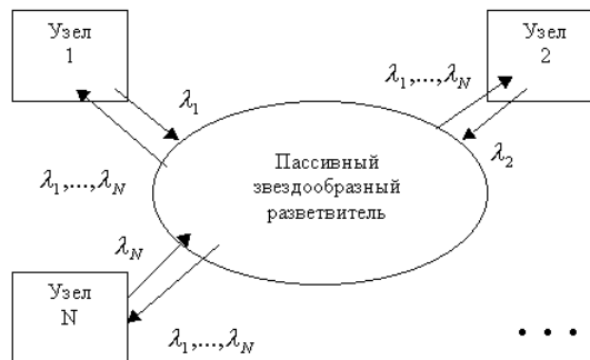
Рис. 19. Модель широковещательной сети ISDN с PON
