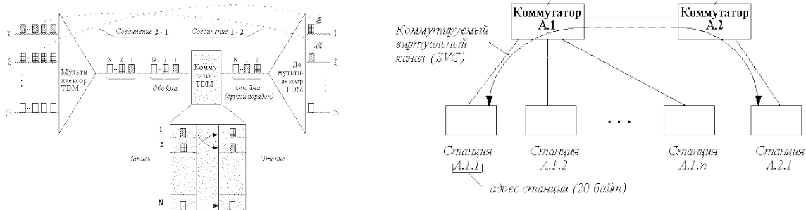
Рис. 5. Принципы построения и коммутации каналов по ATM-технологии [8]
