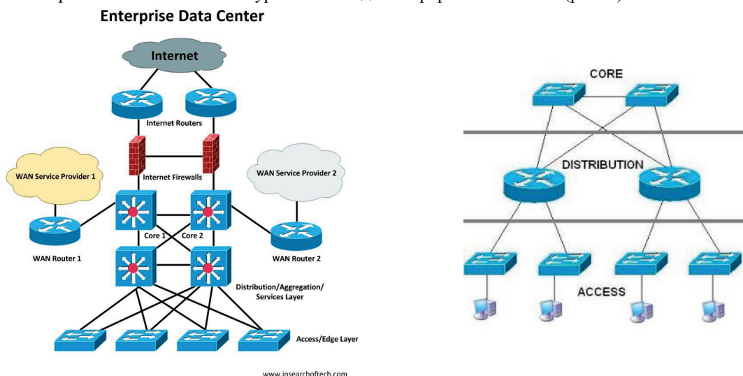
Рис. 1. 3-х уровневая структурная модель иерархической информационной сети: Core-Distribution-Access (CDA) [по классификации Cisco Systems Inc.] [5]
