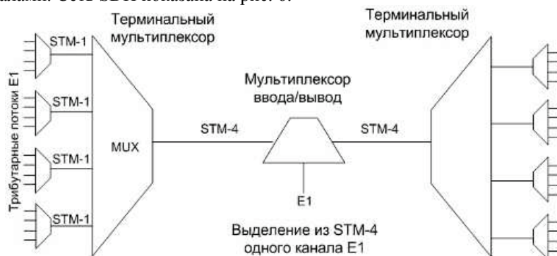
Рис. 6. Пример сети SDH с промежуточным извлечением потока E1 из потока STM-4
