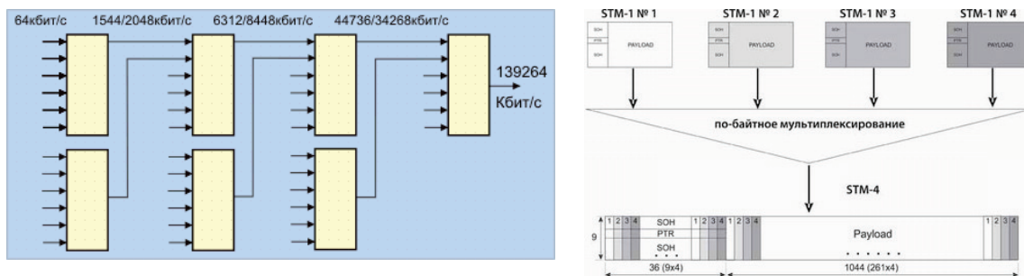
Рис. 7. Схема SDH/PDH-мультиплексирования
