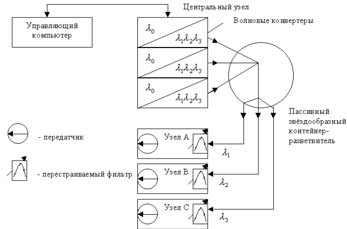
Рис. 21. Модель PON ISDN с коммутацией каналов и пакетов на основе волновых конвертеров
