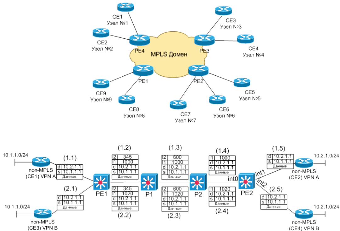
Рис. 8. Схема мережі на базі MPLS-домену і проходження пакета VPN через MPLS-домен [10]
