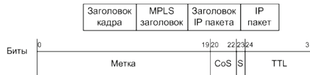
Рис. 9. Место MPLS заголовка в кадре (вверху) та MPLS-метки (внизу)
