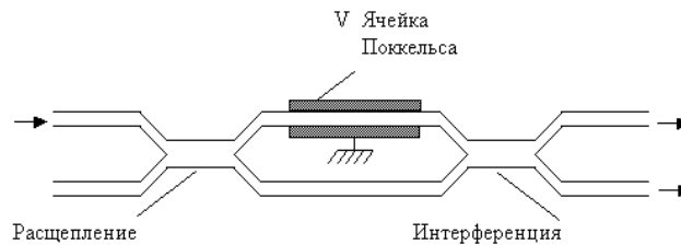
Рис. 17. Двухлучевой оптический разветвитель-коммутатор
