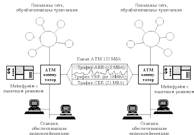
Рис. 4. Совместное использование полосы пропускания классами сервисов ATM
