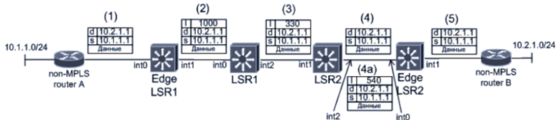
Рис. 11. Пример прохождения пакета через MPLS-домен
