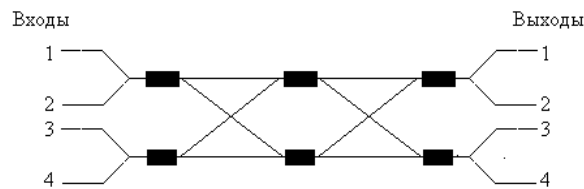
Рис. 18. Схема оптического коммутатора 4 \times 4
