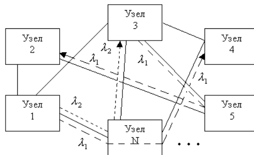
Рис. 20. Модель PON с пассивной волновой маршрутизацией
