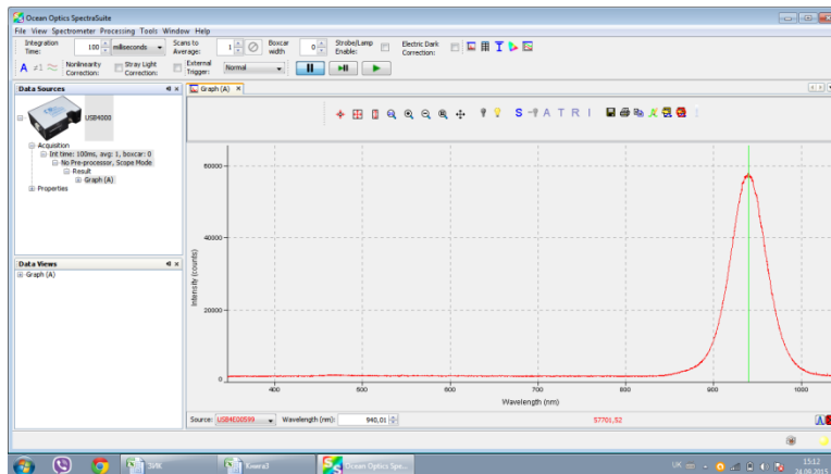
Рисунок 4 – Інфрачервоний спектр.
