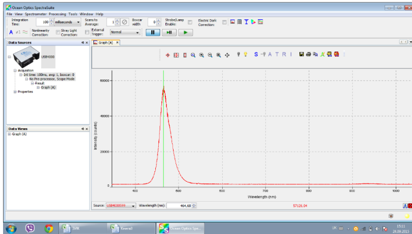
Рисунок 3 – Синій спектр.
